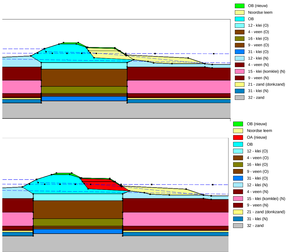
Figuur 5.3 Dijkprofiel benedenrivierengebied II. De Noordse leem (geel) is toegepast in de kern en als steunberm (boven), en alleen in de steunberm (onder). In de ondergrond is een dikke veenlaag aanwezig
