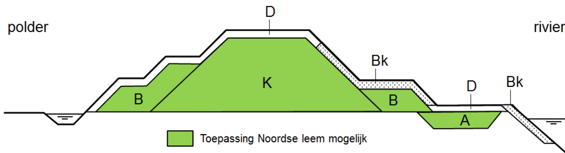
Figuur 4.1 Constructie-onderdelen van een waterkering
