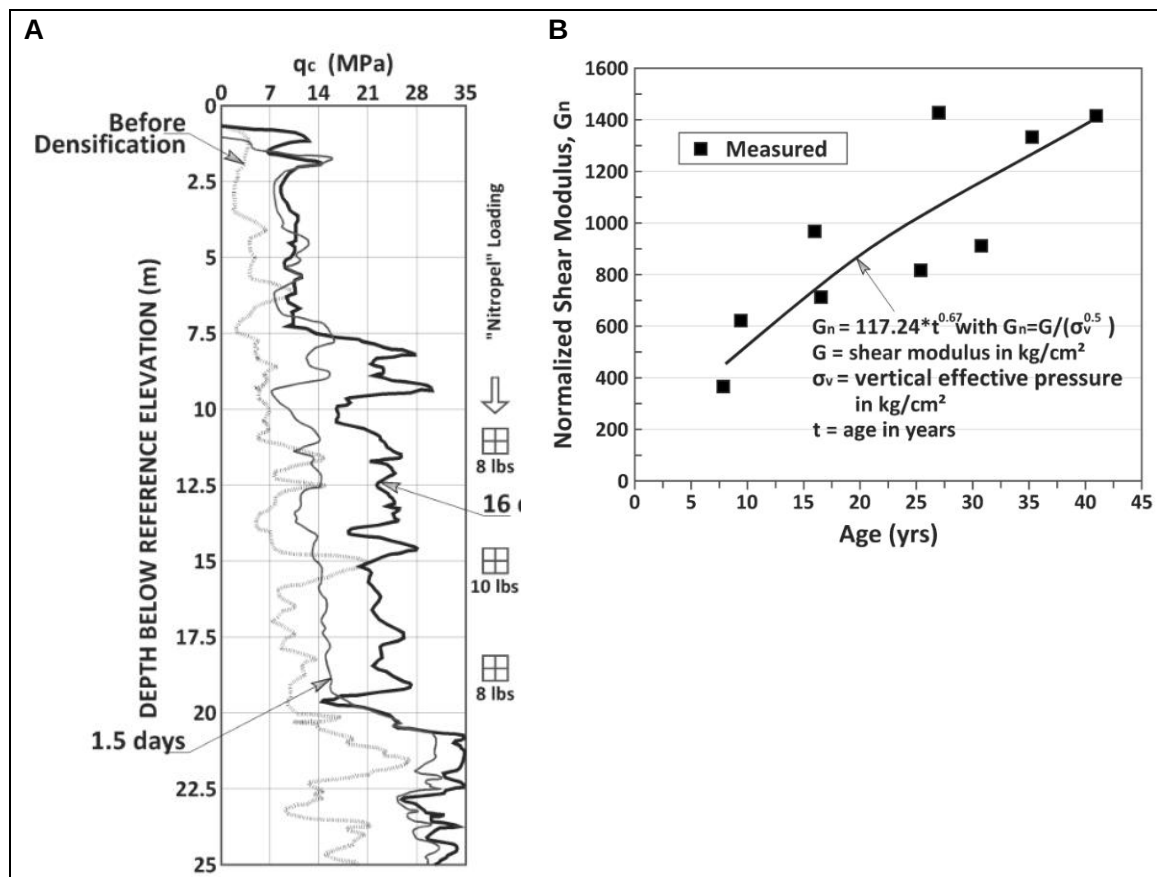
Figuur 3.1 A: Sondeerresultaten die het effect van tijd op korrelcontacten van opgespoten zand illustreren. Na explosieverdichting waarbij de grond verdicht (te zien aan de maaiveld daling), maar de stevigheid afneemt (daling van de conusweerstand, q_c ) door het verbreken van korrelcontacten die in de loop van de tijd waren ontstaan, neemt de sterkte al binnen 16 dagen aanmerkelijk toe (hoge q_c ) door de toename van binding op de korrelcontacten die het korrelskelet verstevigen (uit [33]). B: Toename over de jaren van de schuifstijfheid van fijnkorrelige mine tailings met lage plasticiteit, die net als Noordse Leem het resultaat zijn van het breken van gesteente (uit [33])
