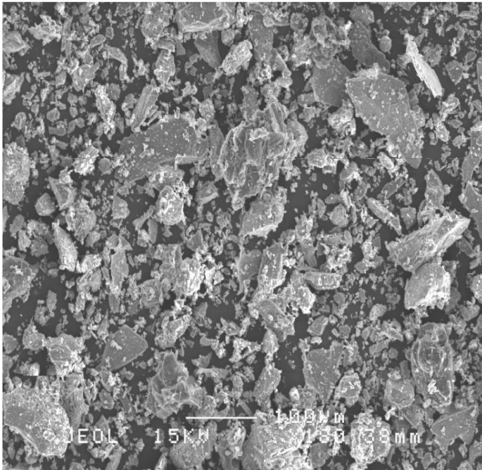
Figuur 3.3 Korrelvorm [13] van Noordse Leem deeltjes zichtbaar in een elektronenmicroscopopname. De witte streep onderaan de SEM opname is 0.1 mm lang, de fijnst zichtbare deeltjes zijn grove lutumdeeltjes (ca 2 \mu m diameter) bij deze vergroting. Het materiaal is zeer hoekig, waarbij opgemerkt wordt dat de zeer fijne minerale deeltjes in natuurlijke grond eveneens zeer hoekig zijn
